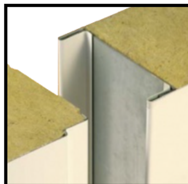
ISOLANT LAINE DE ROCHE
