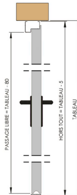
COUPE VERTICALE
